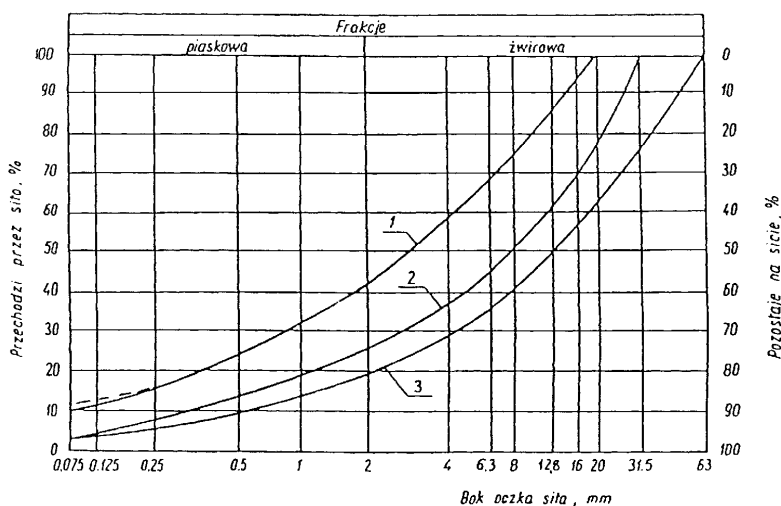
Rysunek 1. Pole dobrego uziarnienia kruszywa
